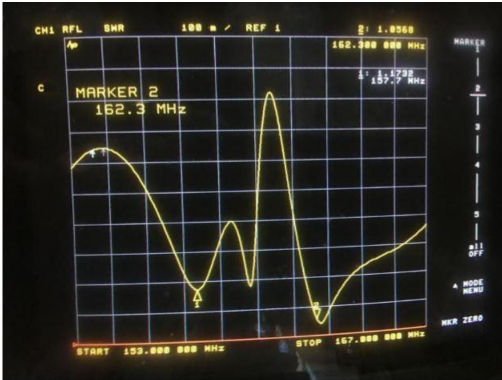
157.700MHz VSWR: 1.173, 162.300MHz VSWR:1.0568
